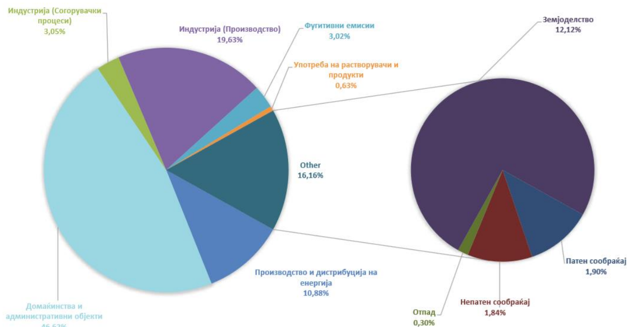
Емисии на PM10 во 2016 година по сектори (извор: Квалитетот на животната средина во РМ - Годишен извештај за 2017)
